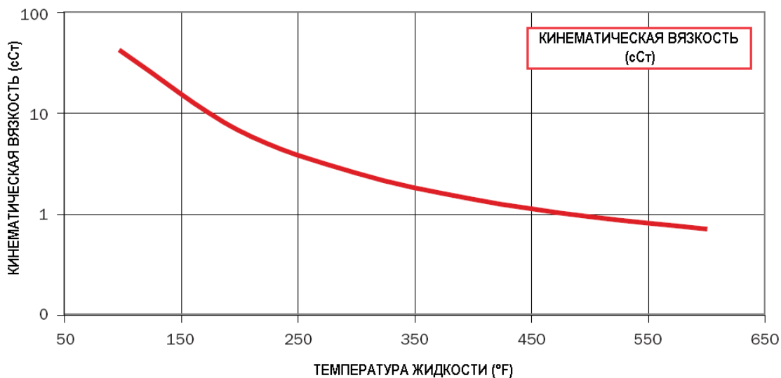
ГРАФИК ЗАВИСИМОСТИ ВЯЗКОСТИ ОТ ТЕМПЕРАТУРЫ RETRO-THERM
